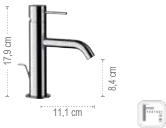
Miscelatore monocomando lavabo. Single-lever basin mixer.
