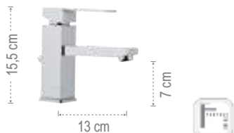
Miscelatore monocomando lavabo. Single-lever basin mixer.
