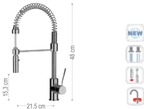
N77E Miscelatore monocomando lavello a molla con doccetta estraibile ed orientabile a due funzioni e cartuccia Ø 35. Spring single-lever sink mixer with pull-out and swivelling 2 functions handshower and Ø 35 mm cartridge.
