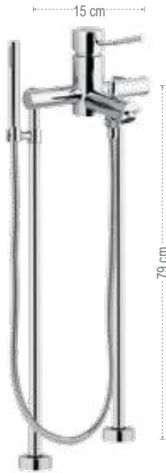
N02XL Gruppo vasca esterno su colonne da pavimento Minimal, con flessibile 150 cm e doccetta ad 1 funzione in ABS anticalcare. Traditional bathtub mixer, on Minimal floor columns, with shower kit, flexible 150 cm with 1 function antilimestone ABS handshower.
