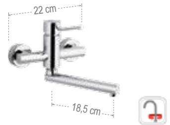
N41 Miscelatore monocomando per lavello a muro, con bocca girevole lunghezza 20 cm. Single-lever wall mounted sink mixer, with swivel spout length 20 cm.
