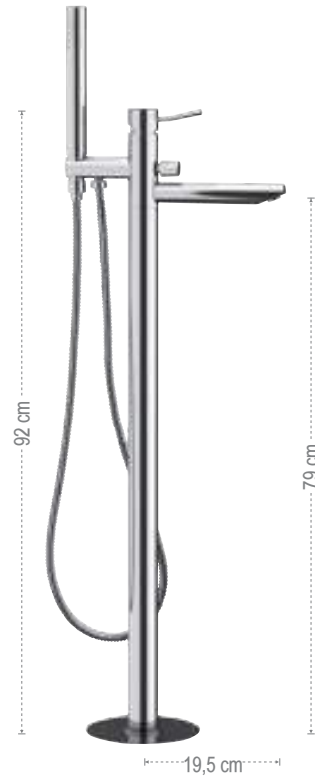
N08 Miscelatore vasca da pavimento con deviatore e kit doccia, senza scarico. Single-lever bath mixer floor mounting with diverter and shower kit.
